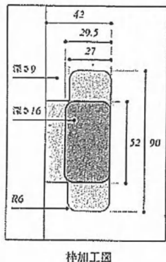
枠加工図
